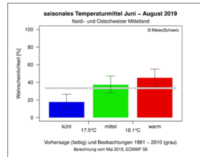
Die Temperaturprognose für den Sommer 2019 von Meteo Schweiz.
