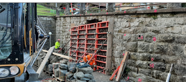
Die Ausbruchstelle wird mit einem Bewehrungsnetz und Filterbeton gesichert
