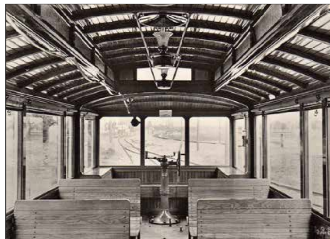
Blick ins Innere des Tramwagens aus dem Jahre 1909 bei der Station Ruderbach
